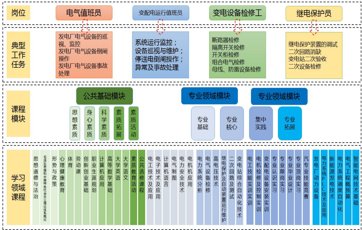
图 1 课程体系图
