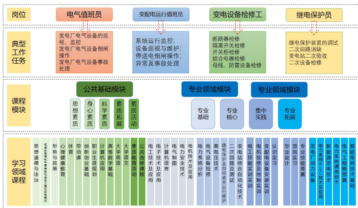
图 1 课程体系图
